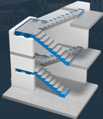
Tronsole - askelääneneristysratkaisut
