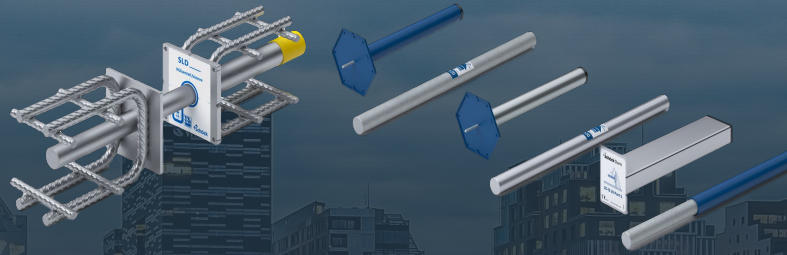
Dorn - liikuntasauvojen vaarnat
