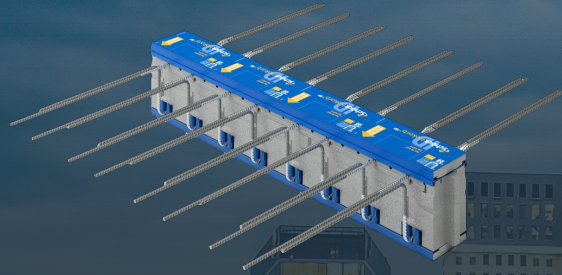
Isokorb - parvekekannattimet
